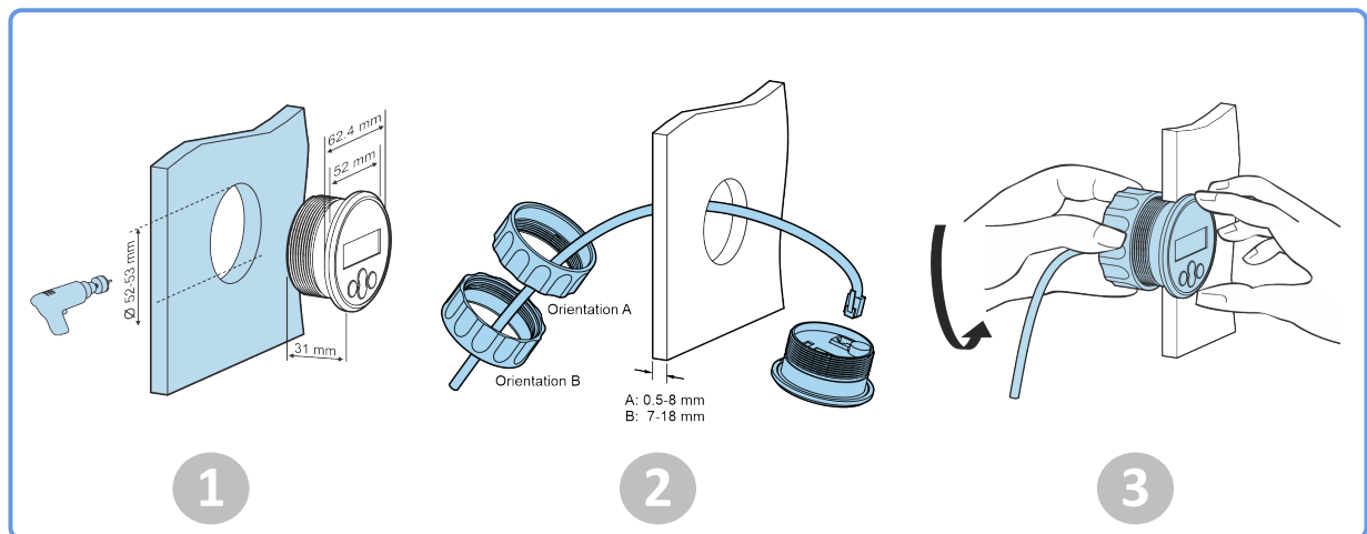
Méthode de montage A.
