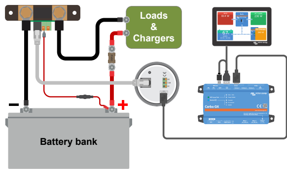
Le contrôleur de batterie est connecté à un Cerbo GX et à un écran GX Touch.
