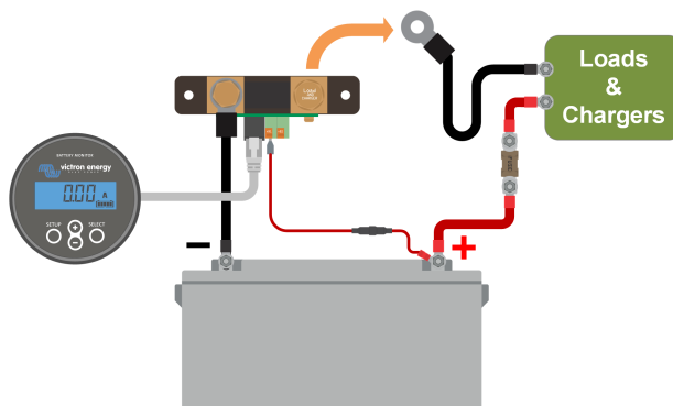
Procédure d'étalonnage de courant nul
