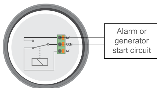
Schéma de câblage interne du contrôleur de batterie avec le relais à l'état hors tension connecté à un circuit externe d'alarme ou de démarrage du générateur.
