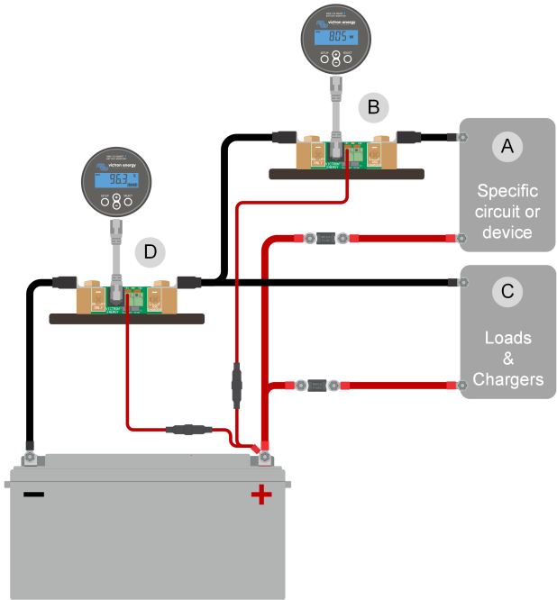
Exemple de câblage pour un système contenant un contrôleur de batterie principal, avec un contrôleur de batterie séparé ayant été configuré comme un compteur CC et supervisant un appareil ou un circuit spécifique. Un contrôleur de batterie est utilisé comme compteur CC (B) et l'autre est utilisé comme contrôleur de batterie (D).
