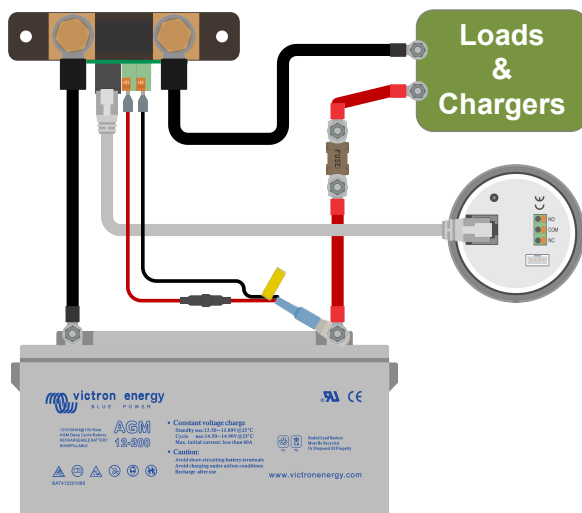
Contrôleur de batterie avec sonde de température d'une batterie auxiliaire.
