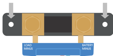
Vue de haut du SmartShunt IP65 montrant les orifices de montage et Vue latérale du SmartShunt indiquant la méthode de montage.
